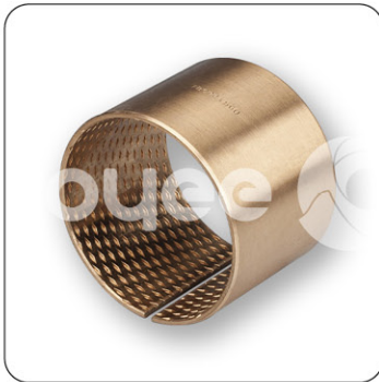
内外倒角 ID and OD chamfers
